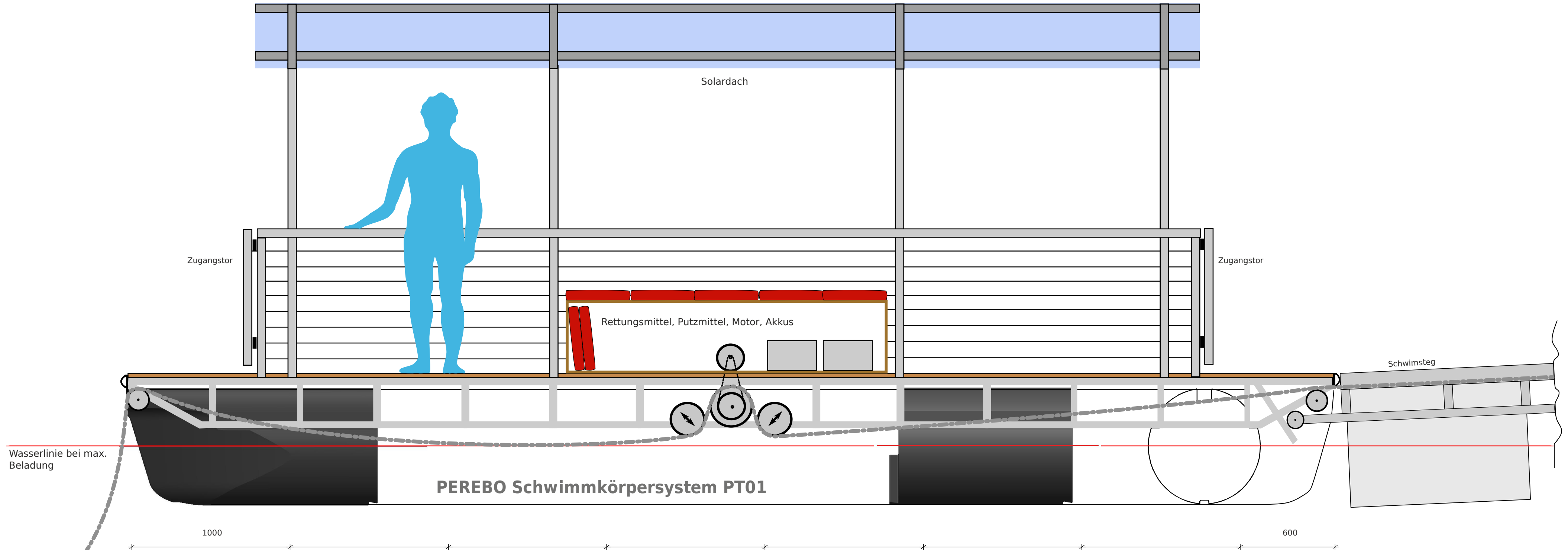
Schematischer Längsschnitt Kettenfähre Scherzligen Thun und Teil Schwimmsteg (Entwurf)
